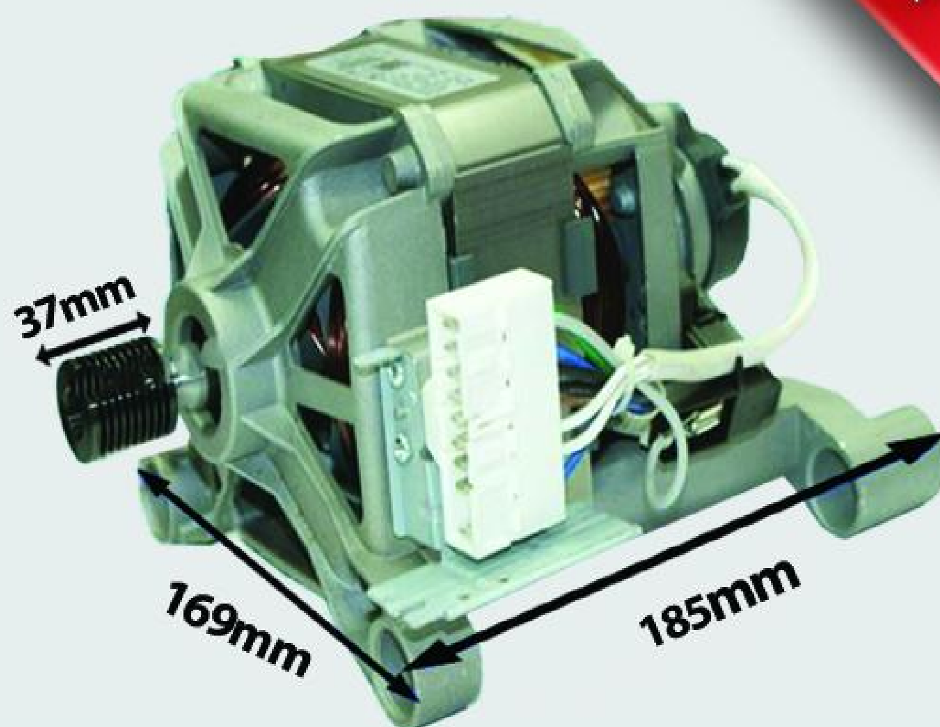
موتور سامسونگ زغالی ۹ فیش
