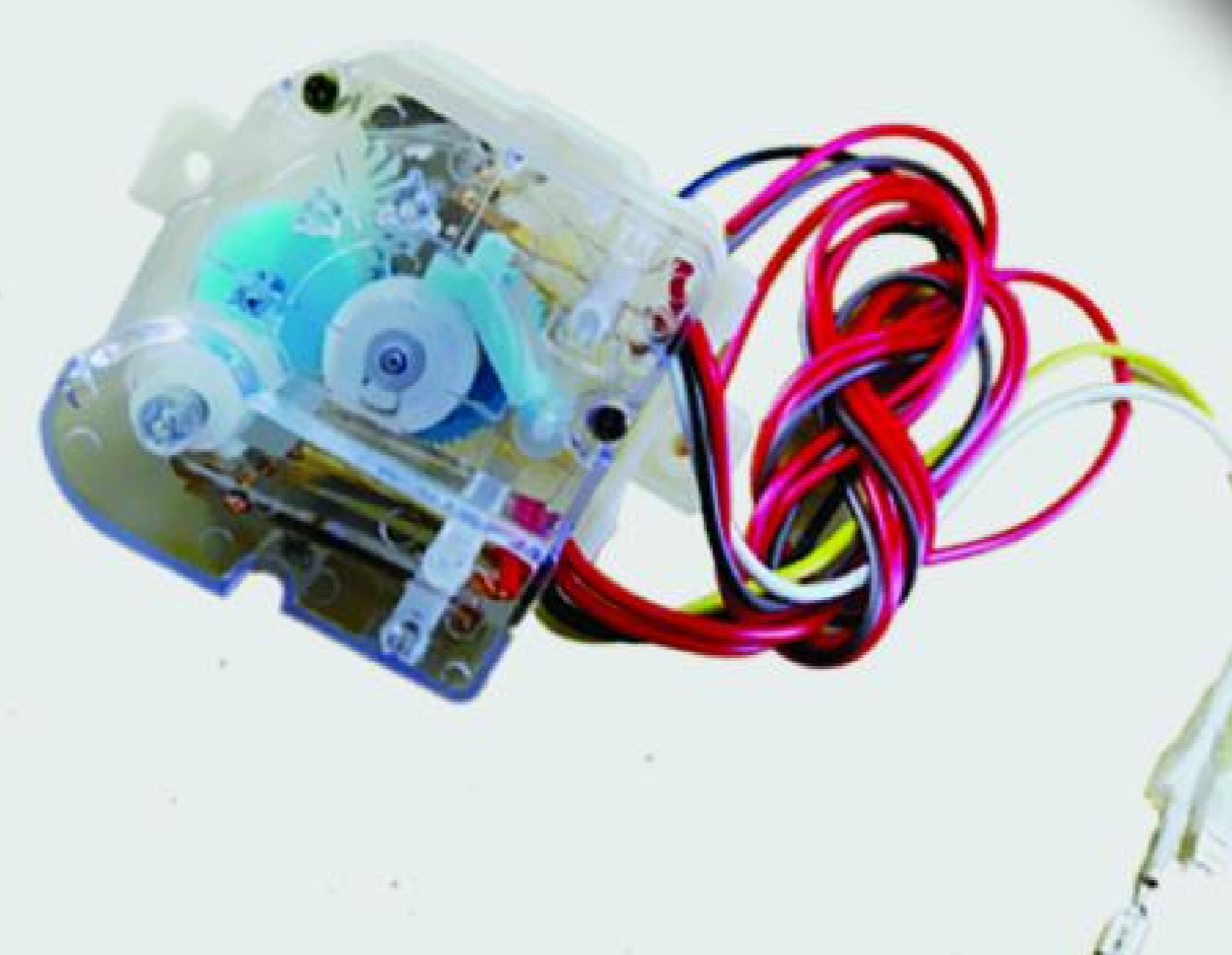
تایمر پاکشوما ۷ سیم
