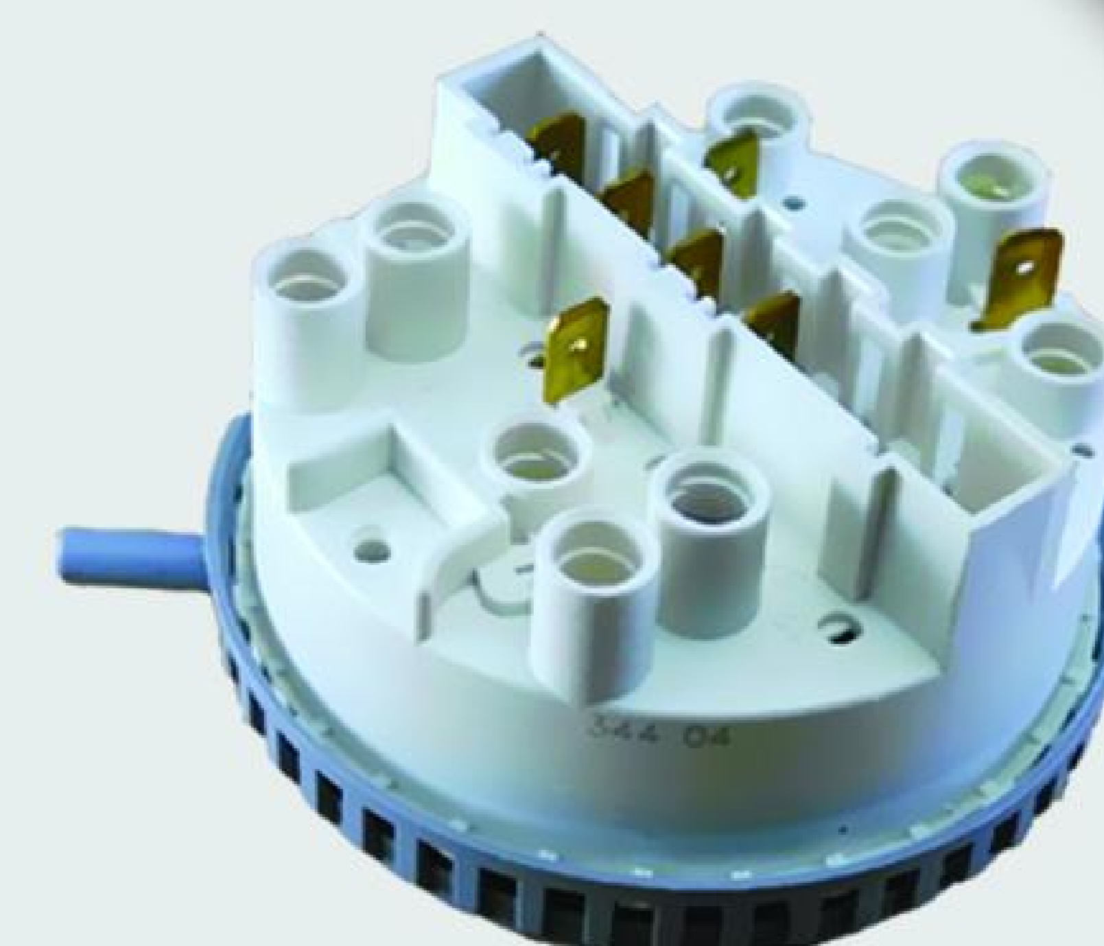
هیدروستات ۷ فیش
