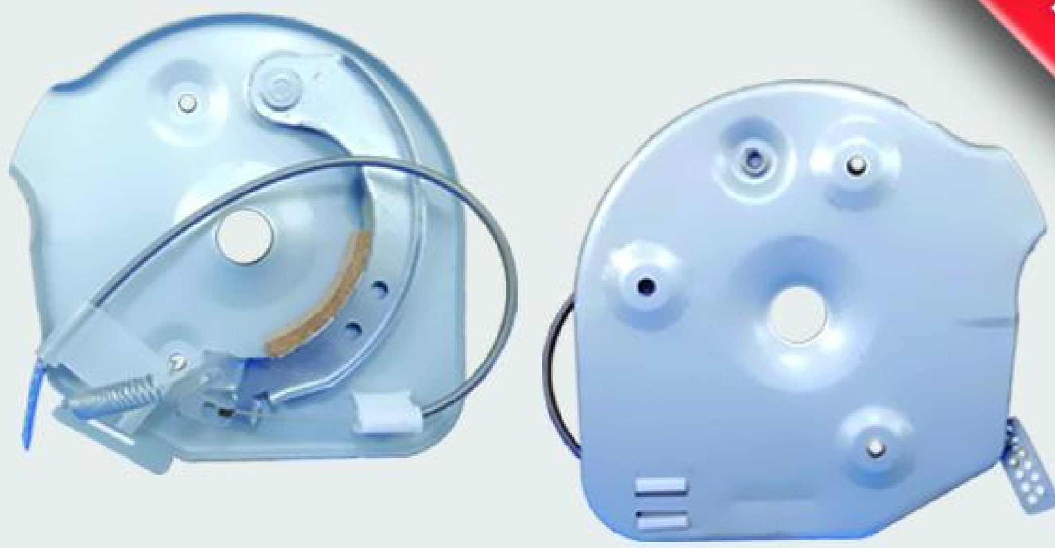
صفحه سیم ترمز هایر
