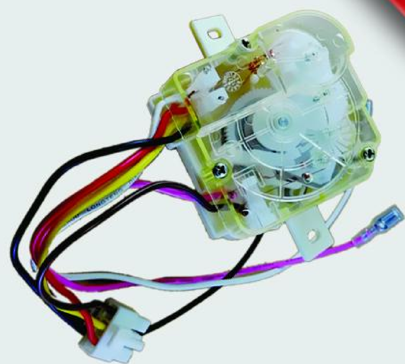
تایمر دوقلو اسنوا ۶ سیم پایه کج
