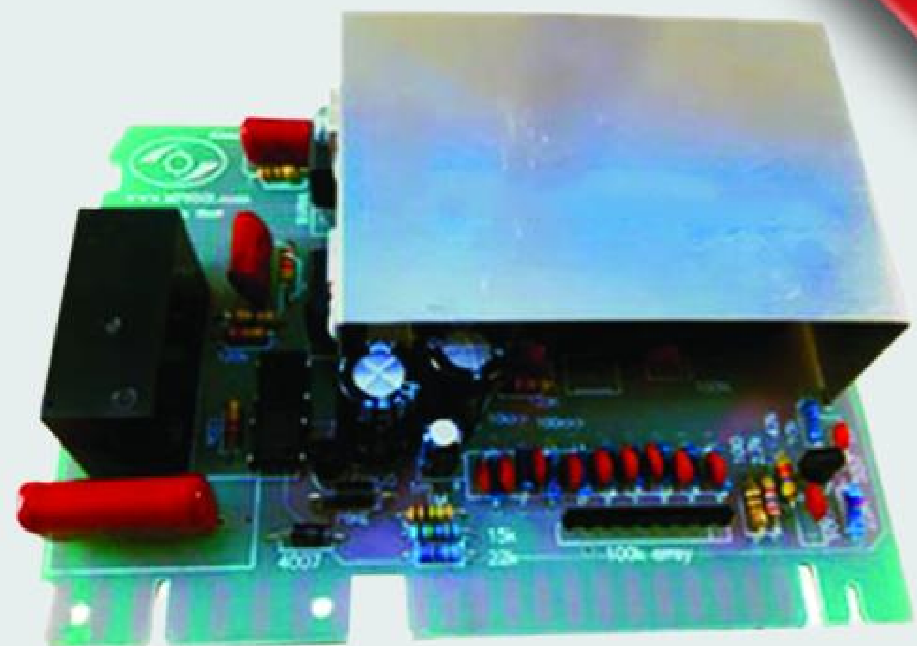
برد آبسال ۷۳۸
